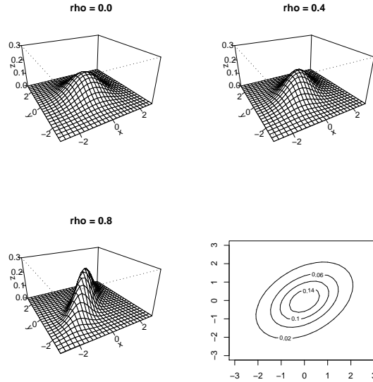
FIGURA 1. Función de densidad de \mathbf{X} \sim N_2(\mathbf{0}, \boldsymbol{\Sigma}) para \rho = 0.0, 0.4 y 0.8 .
